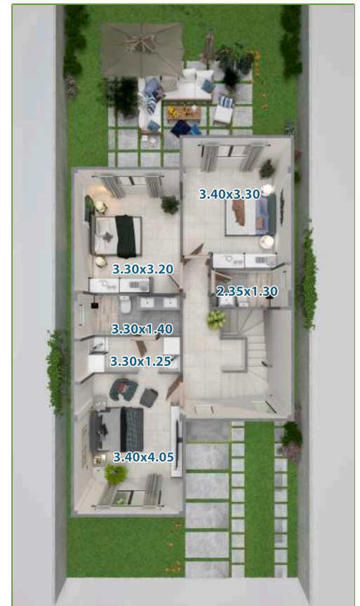
PLANTA ALTA
