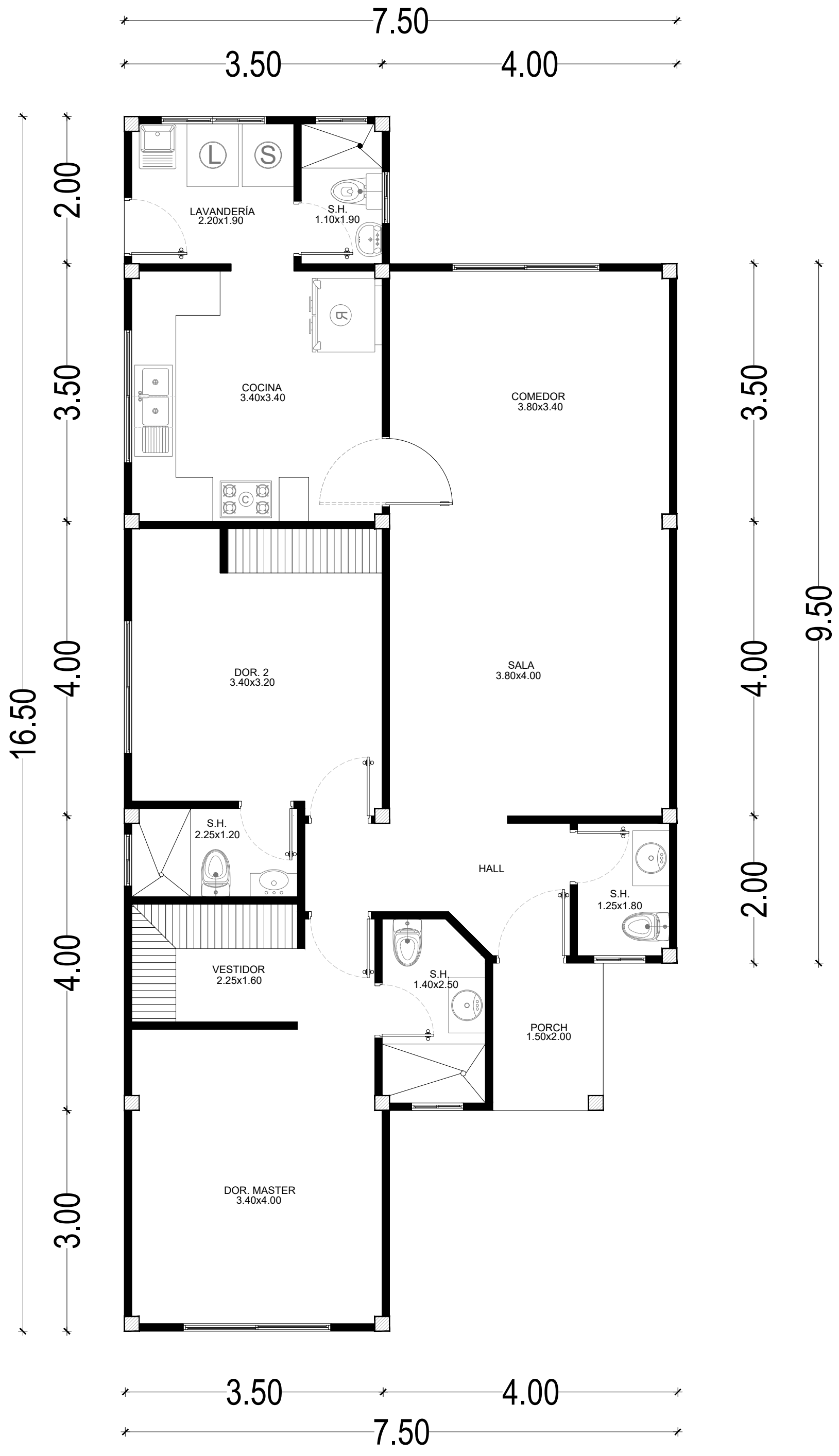
PLANTA
